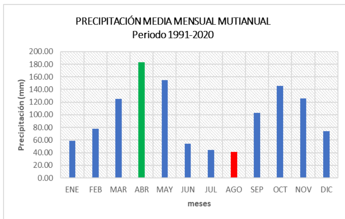
Gráfica 1. Precipitación mensual total multianual periodo 1991 - 2020 municipio de Chaguaní.
