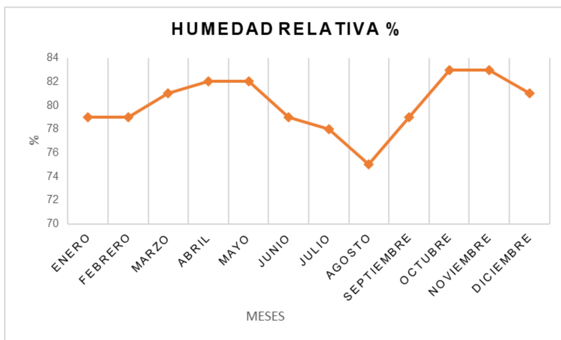
Gráfica 3. Humedad relativa periodo 2010-2024 departamento de Cundinamarca.
